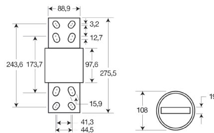
Fig. 3 1200A
