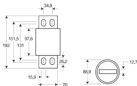
Fig. 2 900A, 1000A
